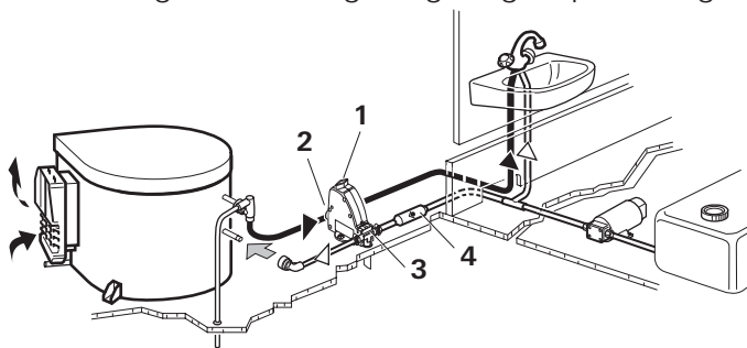
Fig. 3 – monteringsseksempel
